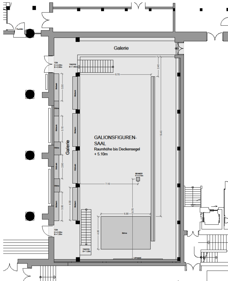
GALIONSFIGURENSAAL ALTONAER MUSEUM M1:100 / DinA 3
